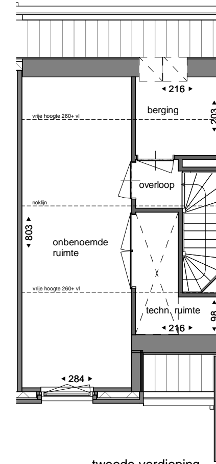
tweede verdieping
