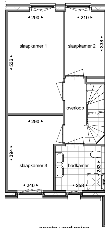
eerste verdieping
